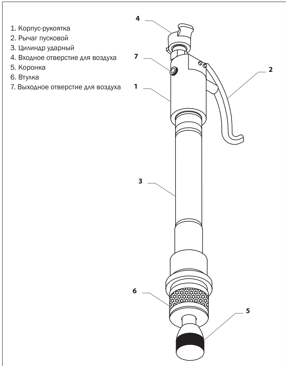
Рис. 2.1 Трамбовки пневматические CPR-3, CPR-5
